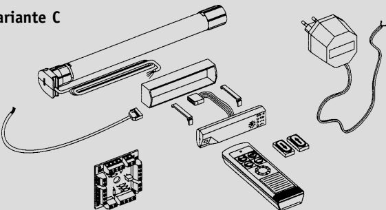
Antriebsmotor, IR-Sender, IR-Empfänger, Steuerkabel 0,5 m, Gruppensteuerungsmodul, Netzteil DC
