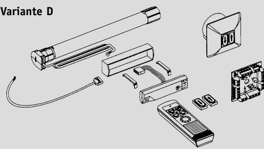
Antriebsmotor, IR-Sender, IR-Empfänger, Steuerkabel 0,5 m, Gruppensteuerungsmodul, Taster mit Trafo
